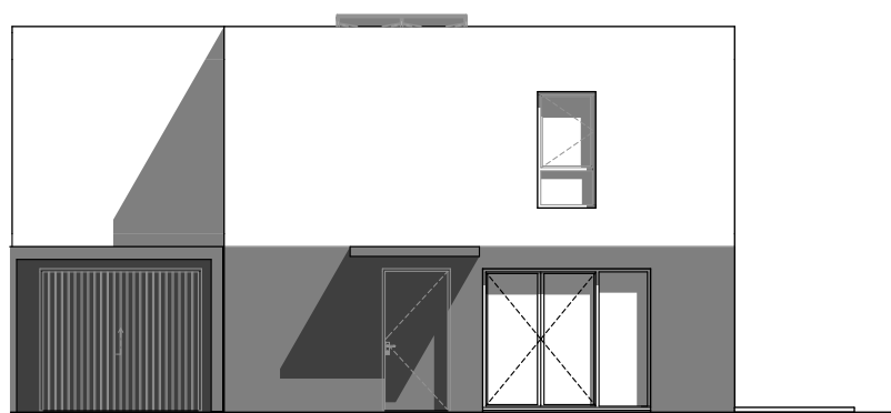
FACADE SUD / EST
