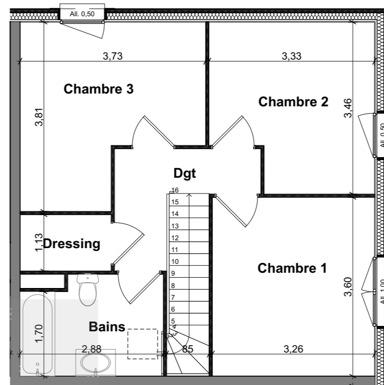
Etage
