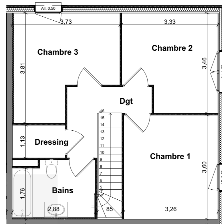
Etage
