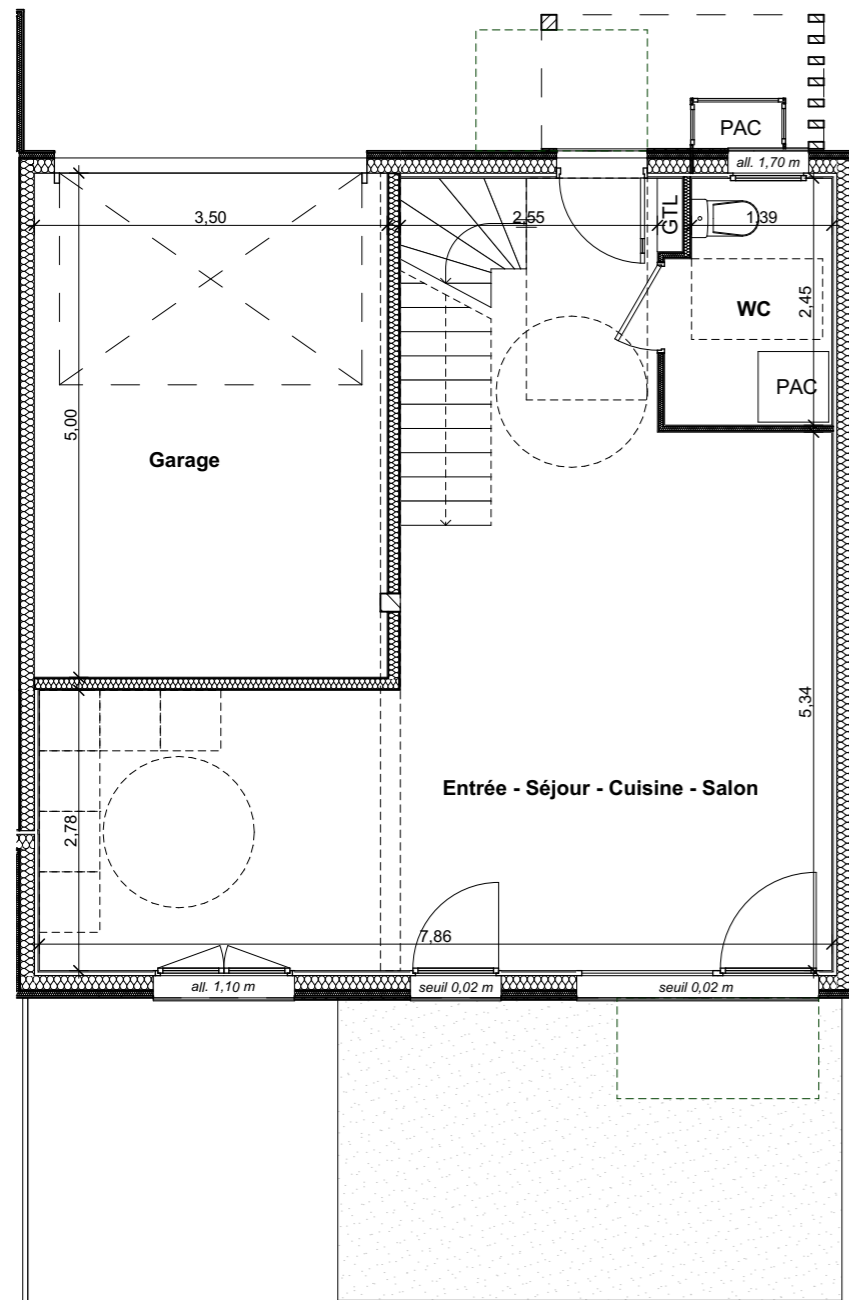
Rez de jardin
