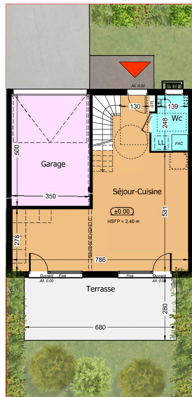
Rez de jardin
